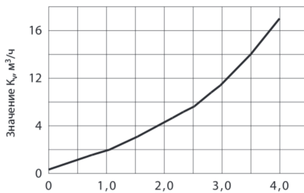
Расходная характеристика
