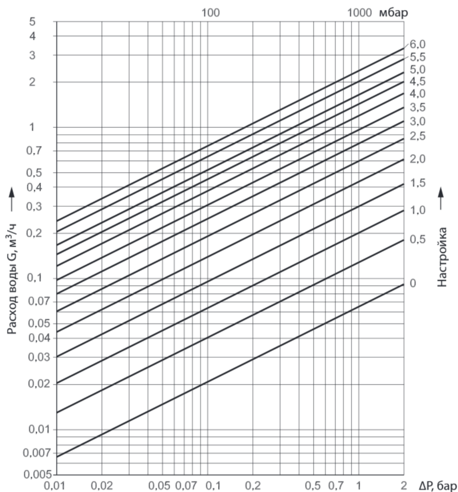
Диаграмма для настройки клапана Leno™ MVT DN = 15 мм LF
