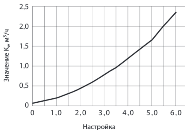
Расходная характеристика
