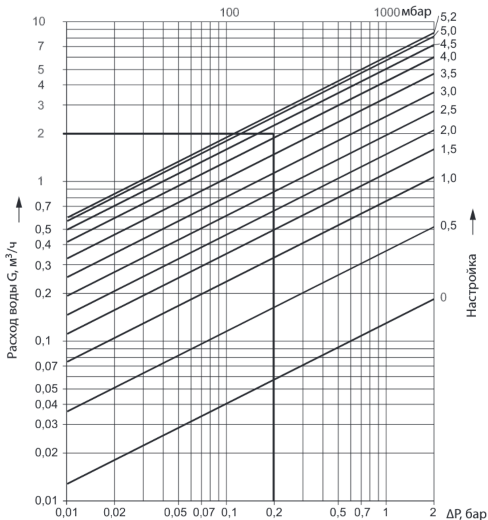
Диаграмма для настройки клапана Leno™ MVT DN = 20 мм
