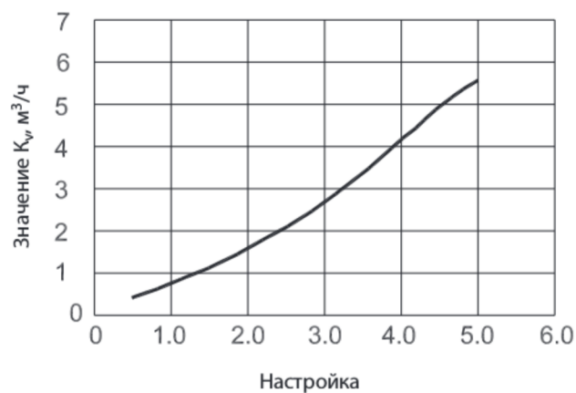
Расходная характеристика
