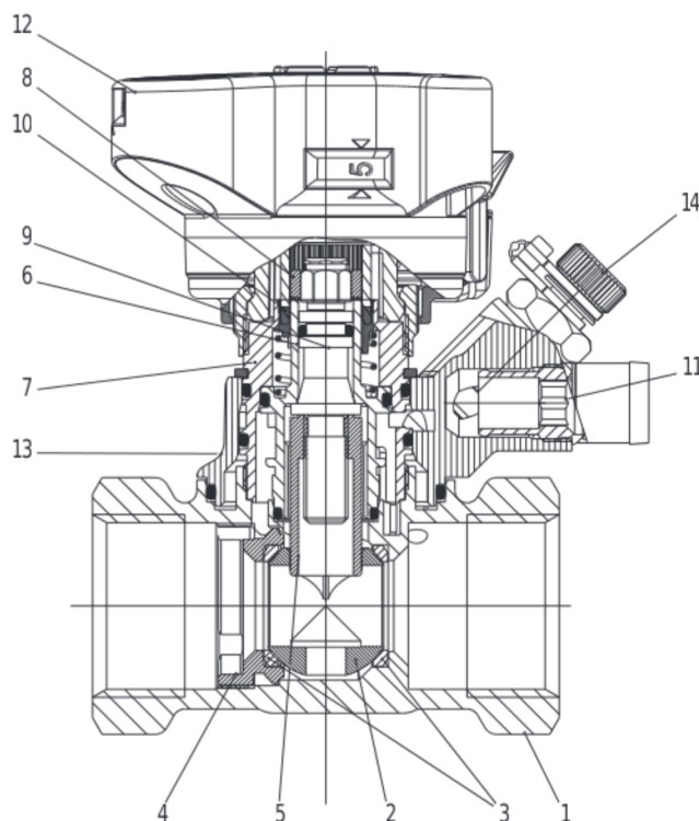
Устройство клапана Leno™ MVT
